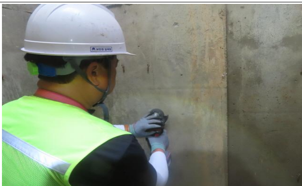
콘크리트 강도시험
